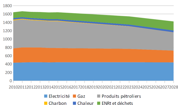
Figure 2-4 : Évolution de la consommation énergétique réelle (2010-2016) et projetée (2017/2028) en France par vecteur énergétique (en TWh) 4
