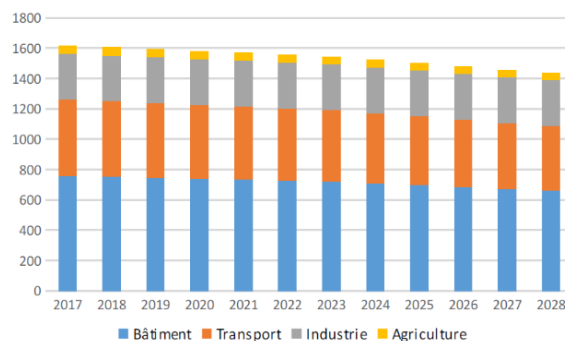
Figure 2-6 : Évolution de la consommation finale d'énergie en France par secteur à partir de 2017 (TWh) 6
