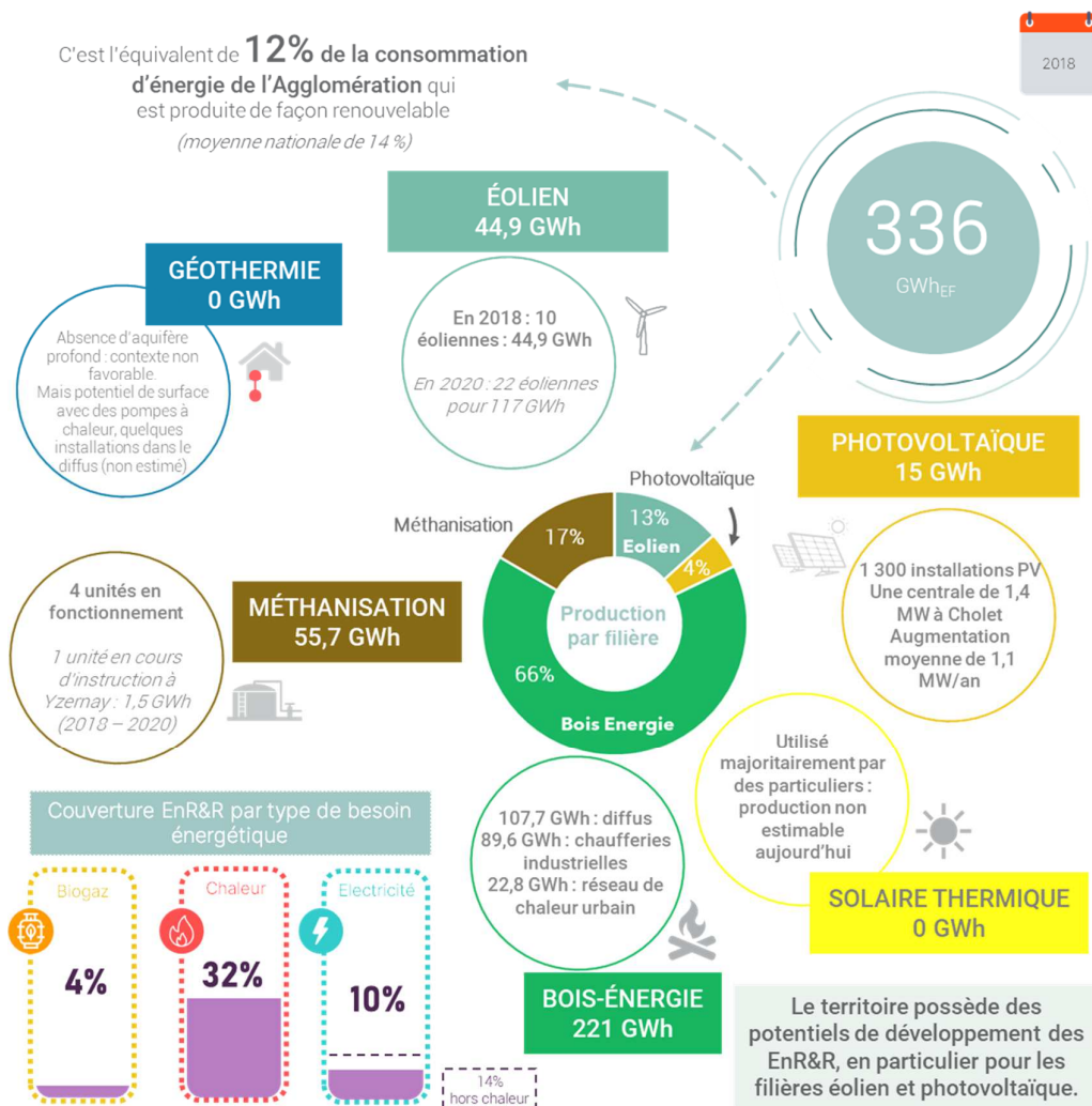
Figure 4-27 : État des lieux des productions d'énergie renouvelable du territoire 27
