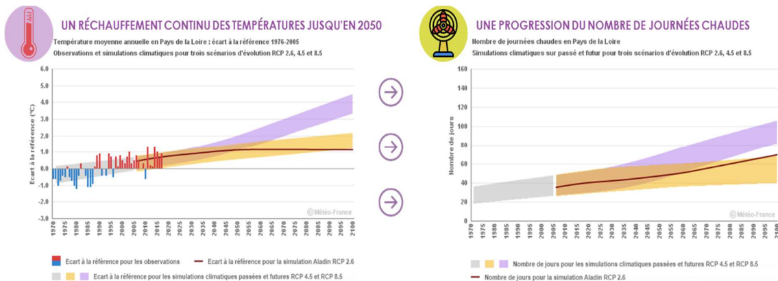
Figure 4-11 : Évolution des températures moyennes et du nombre de jours chauds en région selon les scénarios du GIEC 11
