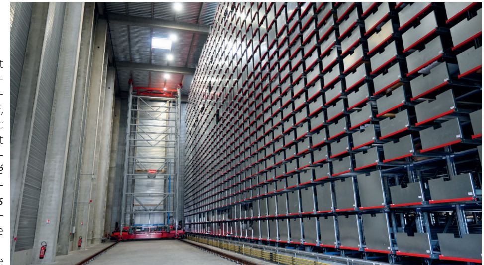
Un transstockeur est un système automatisé constitué de cellules permettant de stocker dans une emprise au sol réduite des éléments tels que des racks de profilés. Chaque cellule peut contenir 1 tonne de charge, soit ici, 1 000 tonnes au total.
