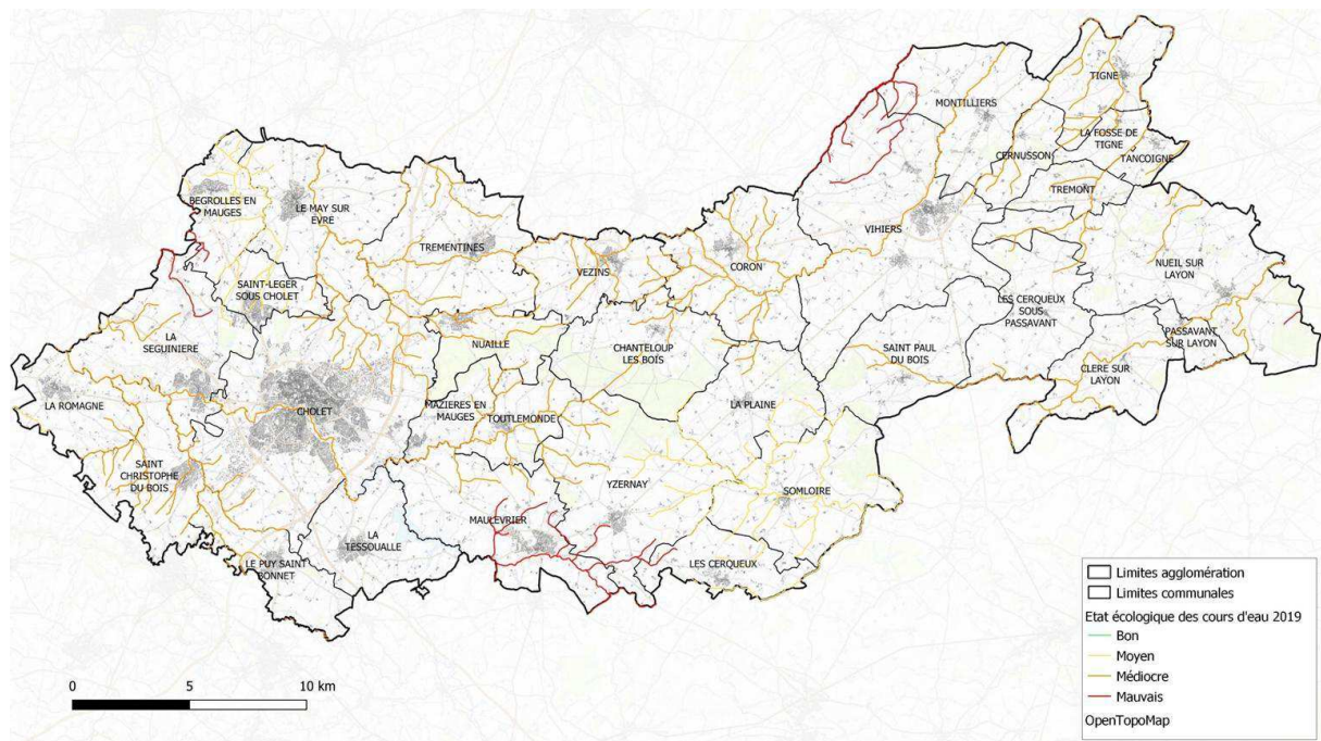
Figure 6: Etat écologique des cours d'eau (état des lieux 2019) présents sur le territoire de Cholet Agglomération
